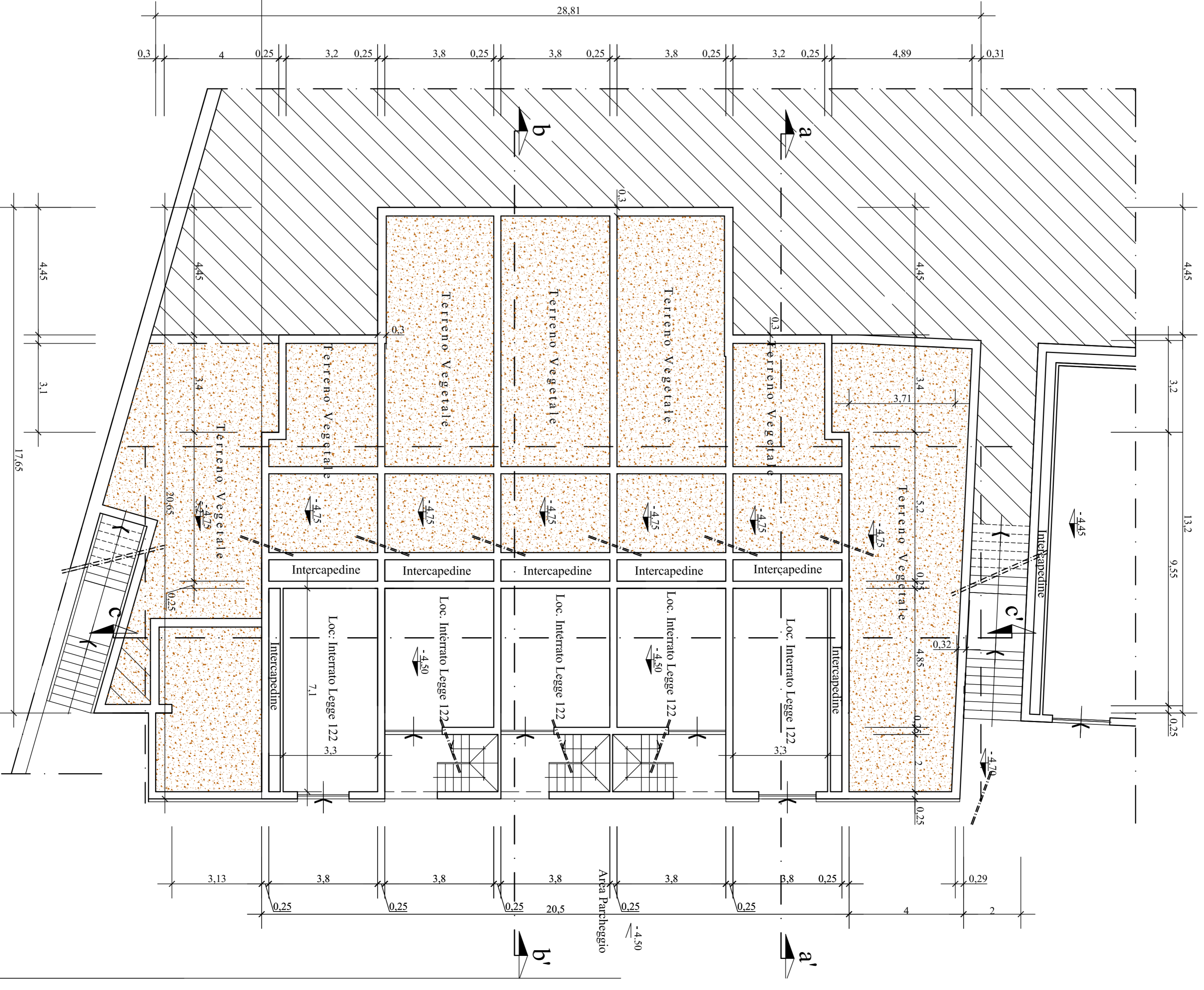
Pianta Piano Fondazione
